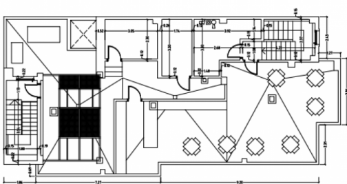
PLANTA CUBIERTA
