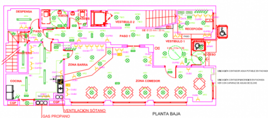
PLANTA BAJA
