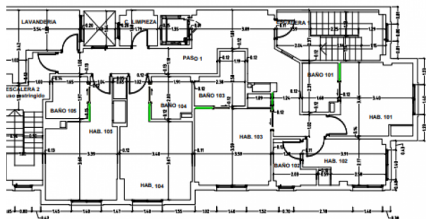
PLANTA 1ª
